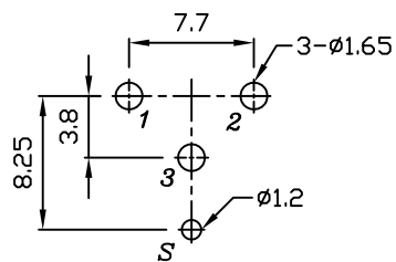
P.C.B LAYOUT(±0.1) (BOTTOM VIEW)
