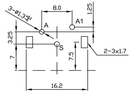
P.C.B LAYOUT(±0.1) (BOTTOM VIEW)
